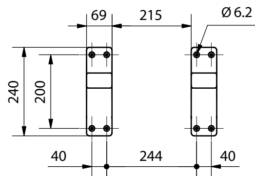
Detalle fijaciones (1:10)
