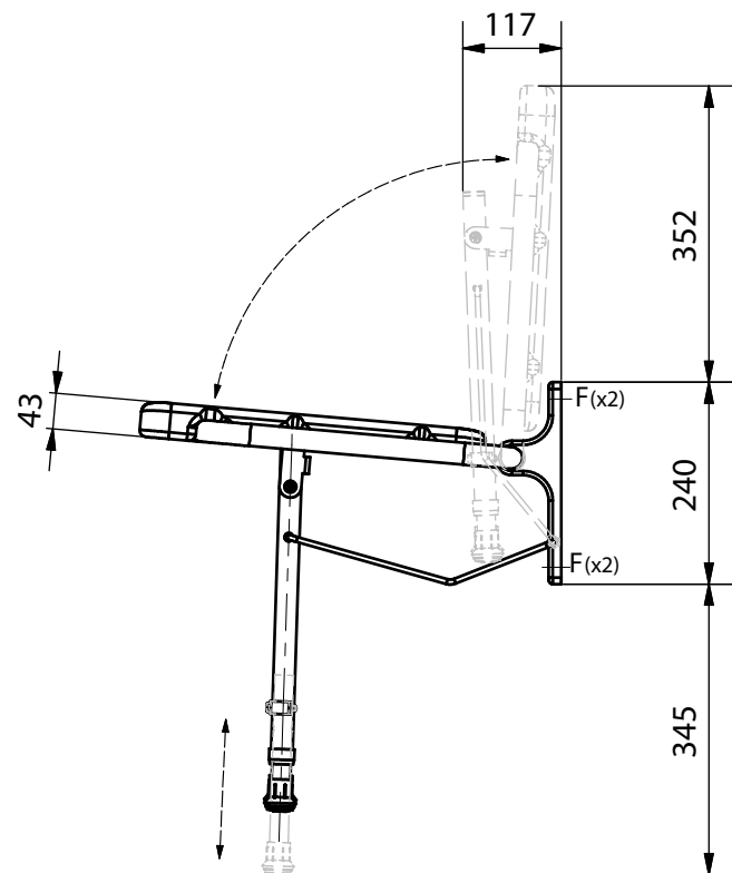
Detalle fijaciones (1:10)
